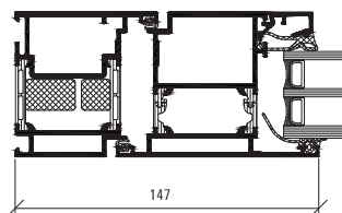
Horizontalsnitt Profilmått, skala 1:4
