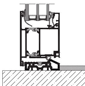
Anslutningsprincip, skala 1:4
