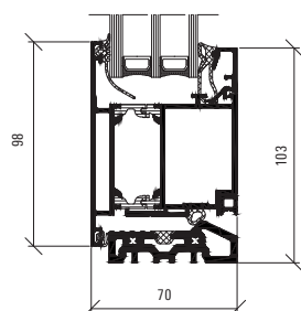
Vertikalsnitt Profilmått, skala 1:4
