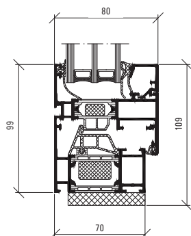
Profilmått öppningsbart fönster, skala 1:4
