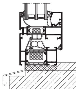
Anslutningsprincip öppningsbart fönster, skala 1:4
