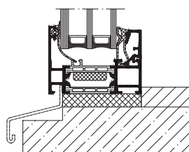
Anslutningsprincip fast fönster, skala 1:4
