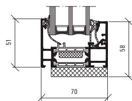
Profilmått fast fönster, skala 1:4
