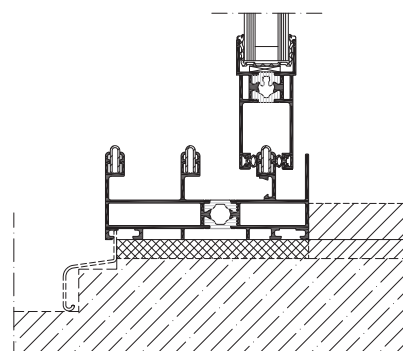
Anslutningsprincip 3-spårs skjutparti, skala 1:4
