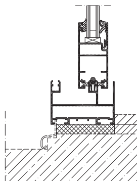
Anslutningsprincip 2-spårs skjutparti, skala 1:4
