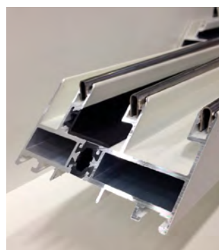
Karm Schüco ASS 32 med bruten köldbrygga.
