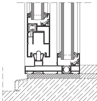
Anslutningsprincip, skala 1:4
