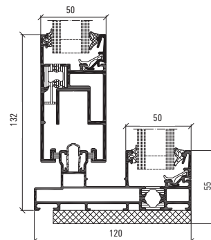
Skjutparti dubbelglas, skala 1:4
