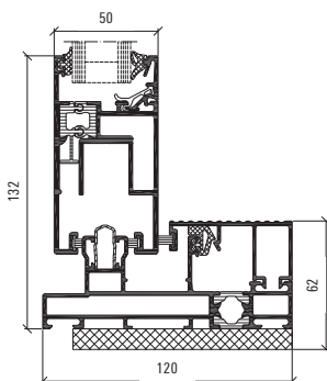
Skjutparti med tröskel, skala 1:4
