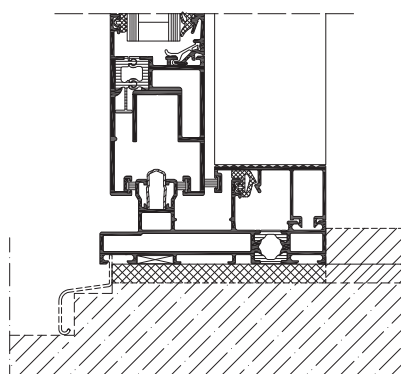
Anslutningsprincip, skala 1:4
